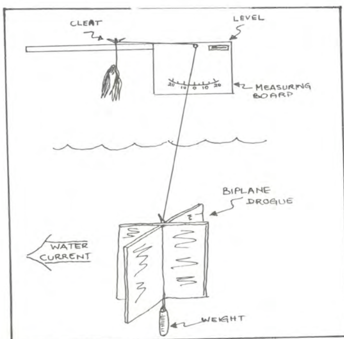
Fig. 10-15: Bi Plane Drogue.
